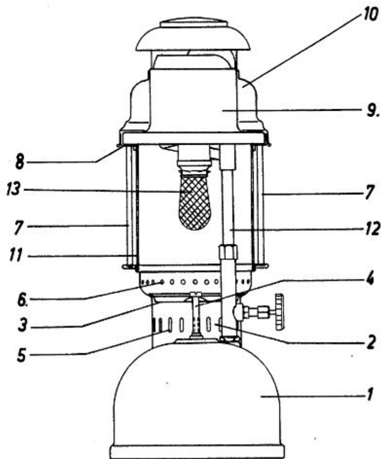
Le croquis du brevet DE728350
